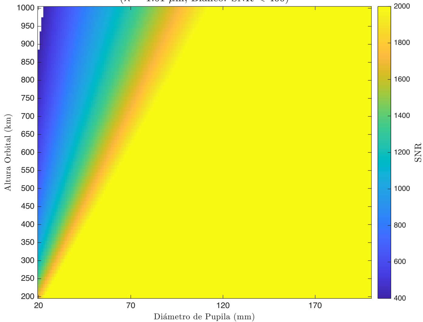
SNR - Cassegrain - Detector 2 ( \lambda = 1.61 \mu\text{m} , Blanco: SNR < 400)
